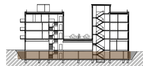
Řez A
