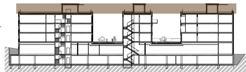
Řez B
