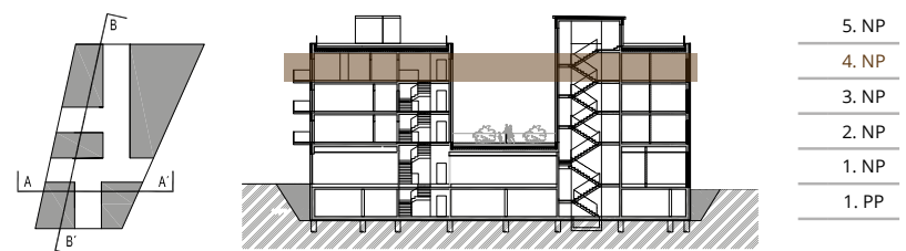
Řez A
